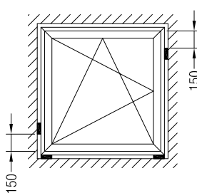
Поворотно- откидное окно
