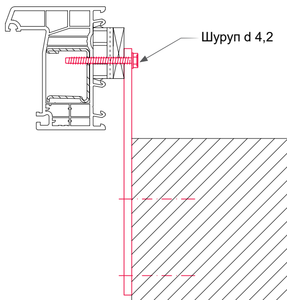
Консоль
