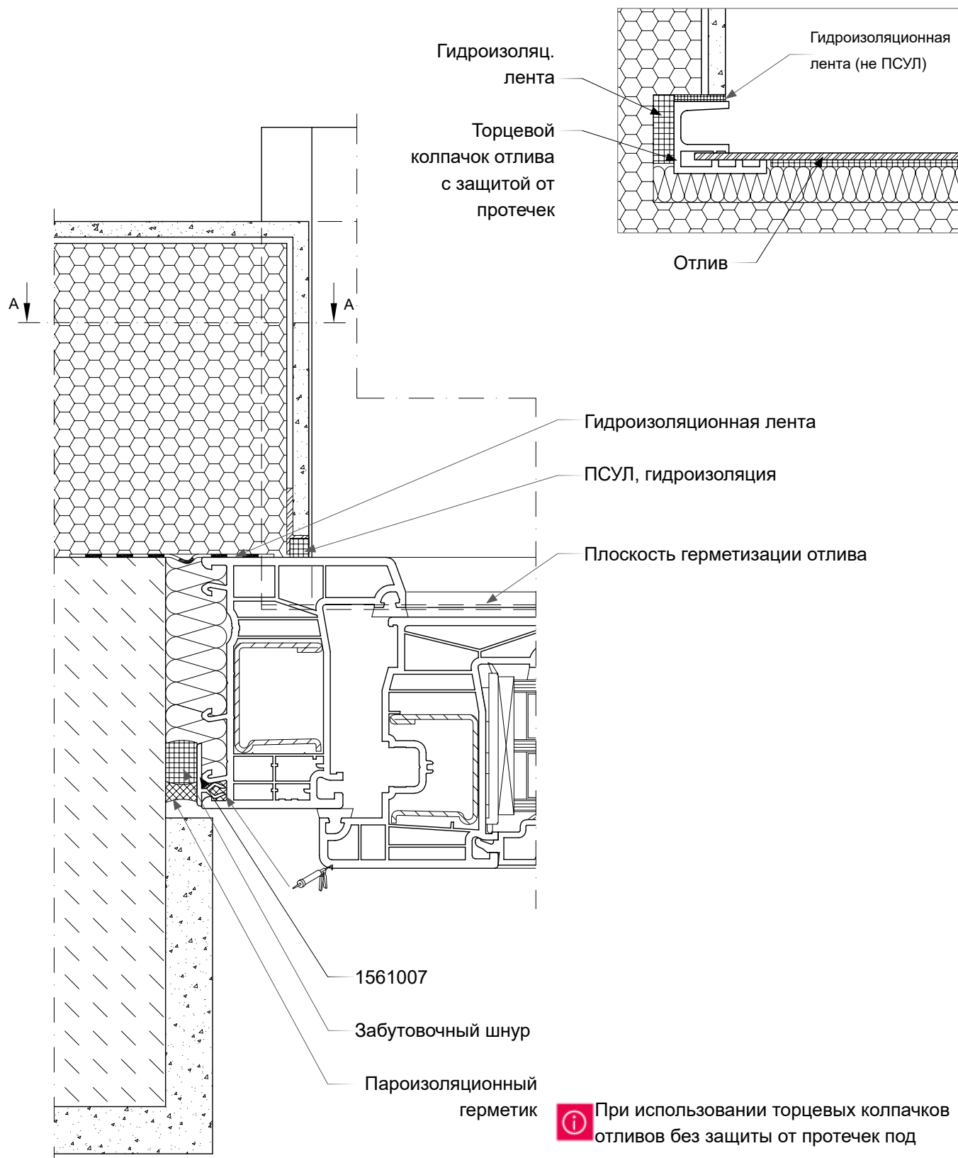
Сечение А-А:
