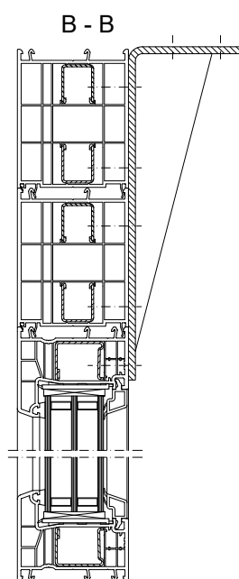
Рис. 18: Крепление доборного профиля
