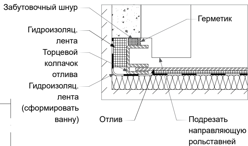
Сечение А-А:
