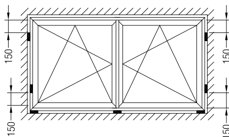
Двустворчатые окна без импостов (колодка в середине нижнего бруска коробки не должна влиять на функциональность окна)
