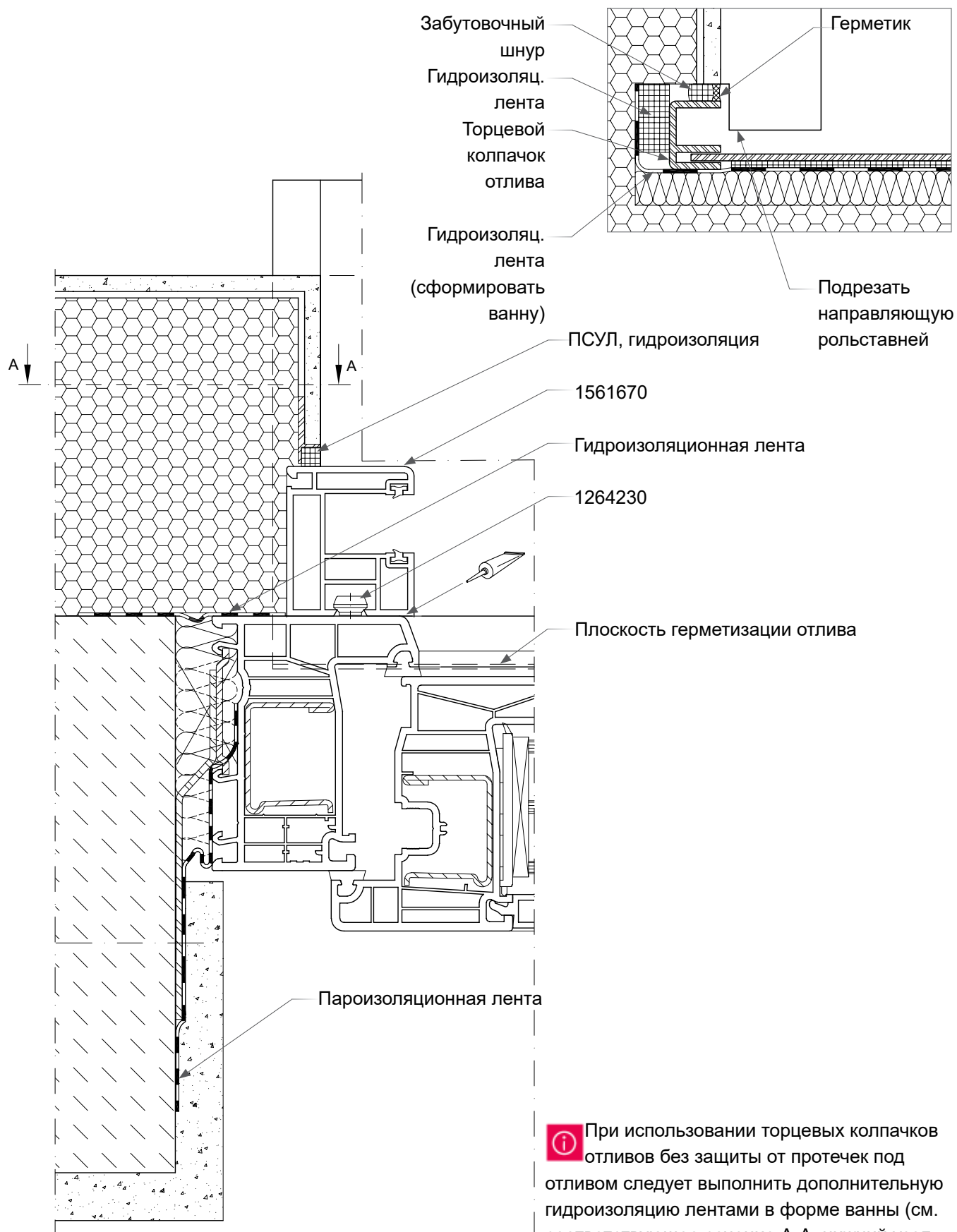
Сечение А-А:
