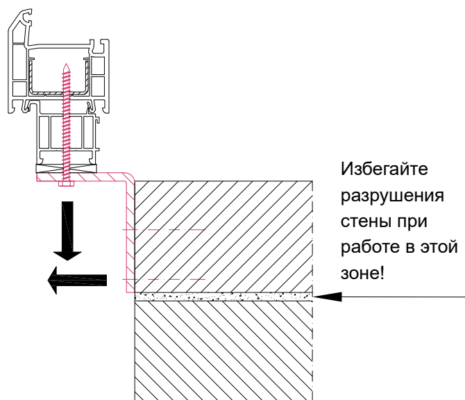
Уголок
