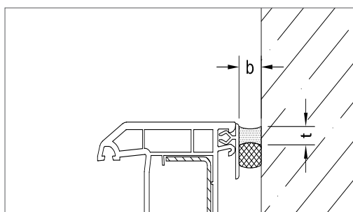
Рис. 23: Соотношение размеров слоя обмазочных герметиков в монтажных швах
