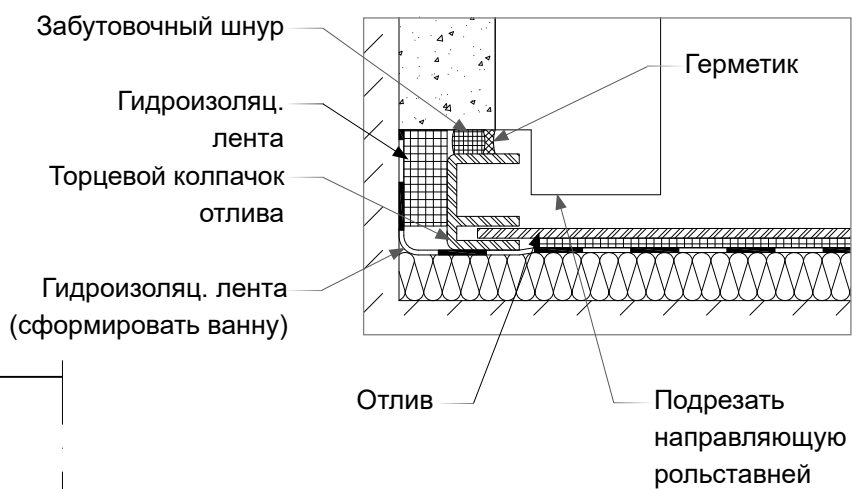
Сечение А-А:
