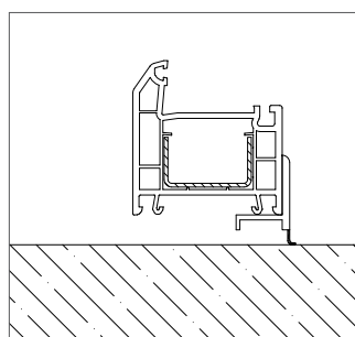
ПСУЛ пароизоляционные
