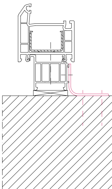
Уголок
