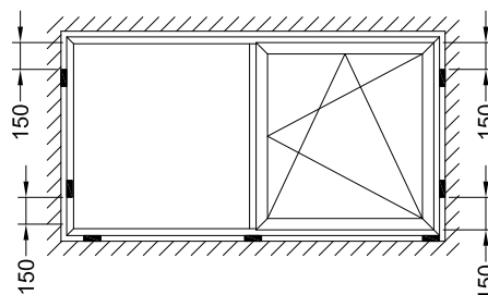
Окна с поворотно-откидными (поворотными) створками и глухой частью
