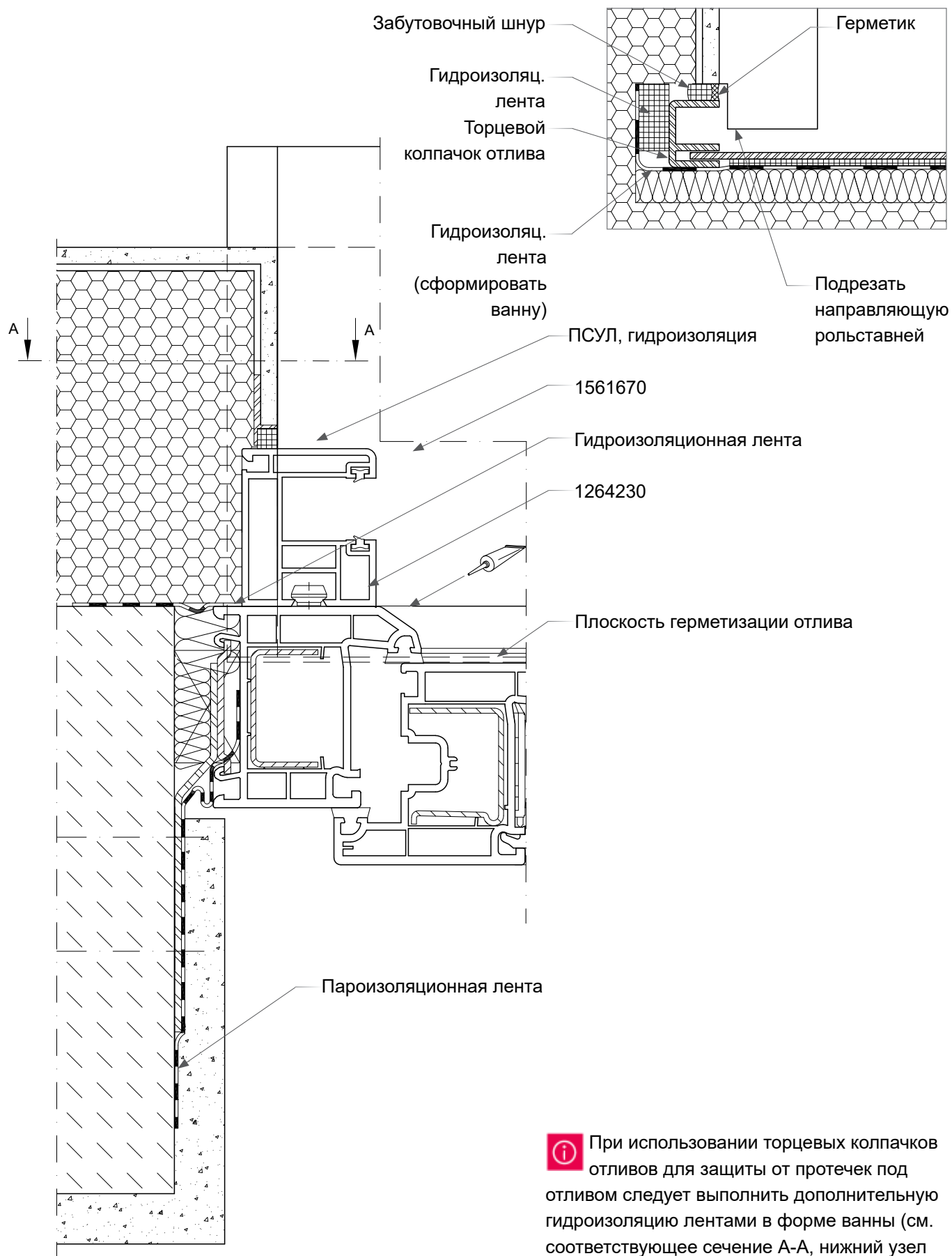
Сечение А-А:
