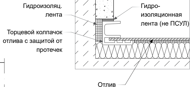
Сечение А-А:
