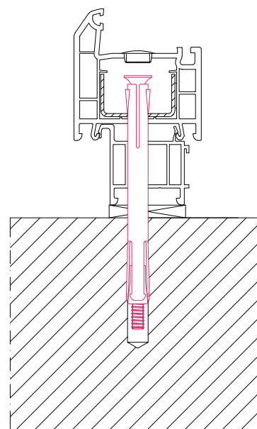
Дюбель
