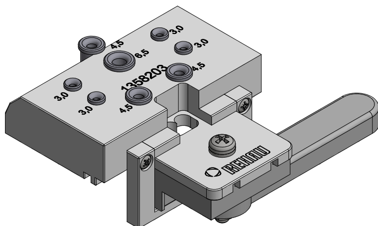
Шаблон для установки мех. соединителей INTELIO
