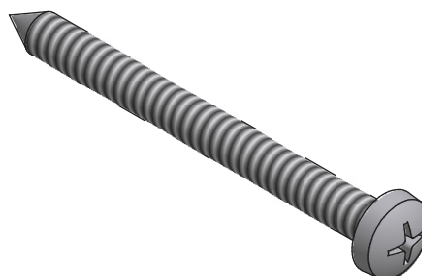
Шуруп 6,3 x 70 (ISO 7049), сталь оцинкованная
