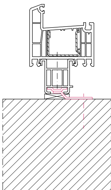
Монтажная (анкерная) пластина
