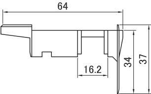
3510 + 3511 Штульповый колпачок
